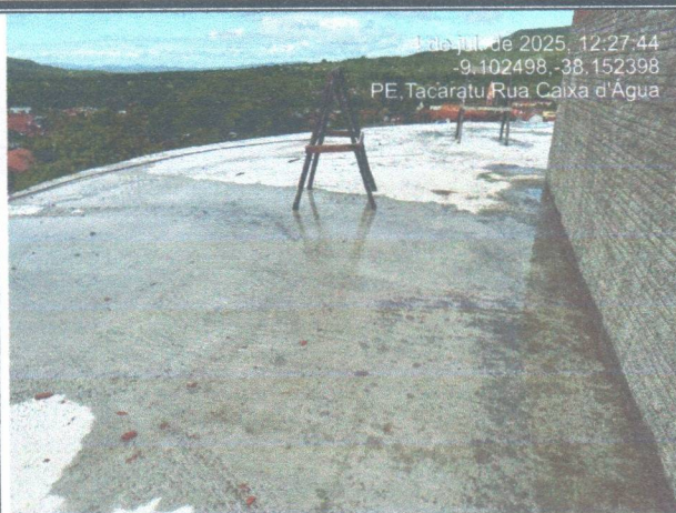
Foto 1: LAJE CONCRETADA EM CURA
